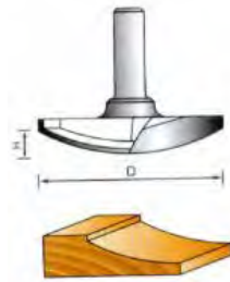
WAVE 波板専用
